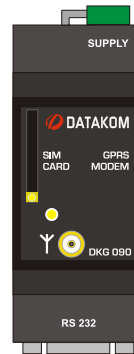
GPRS MODEM
